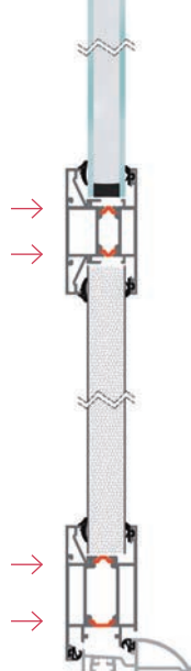
Profilés à double feuillure et rupture de pont thermique
