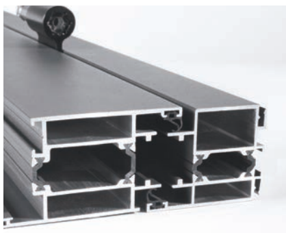
Profilés à double feuillure et rupture de pont thermique
