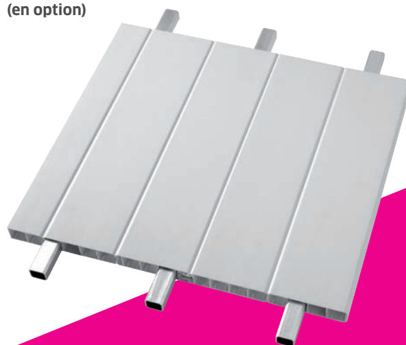
Renfort aluminium dans les panneaux (en option)
